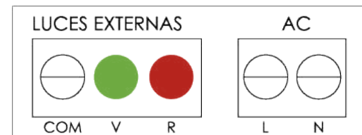
Diagrama de conexiones
